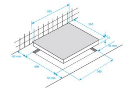
Schéma d'encastrement
